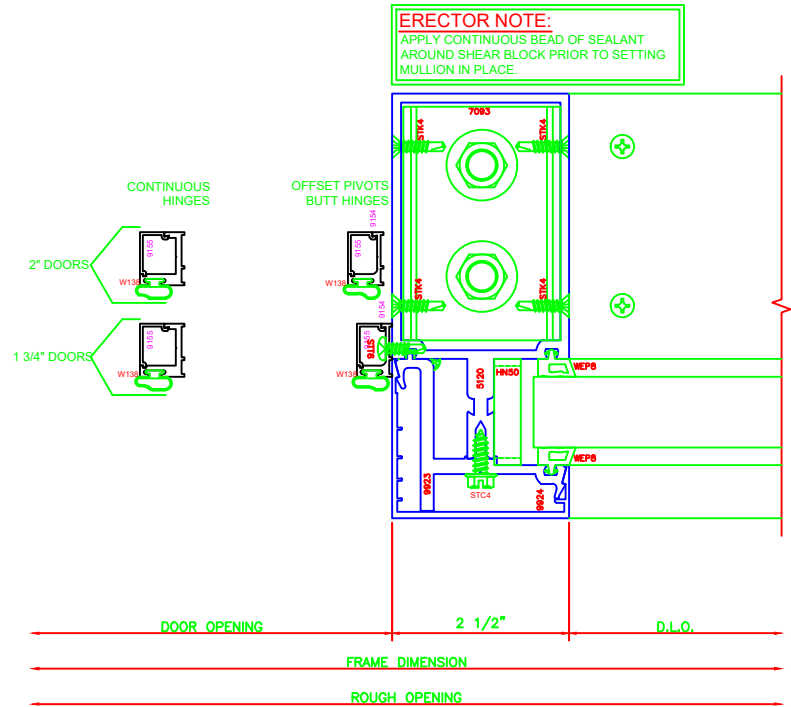
823 O.G. JAMB 5600 6"
