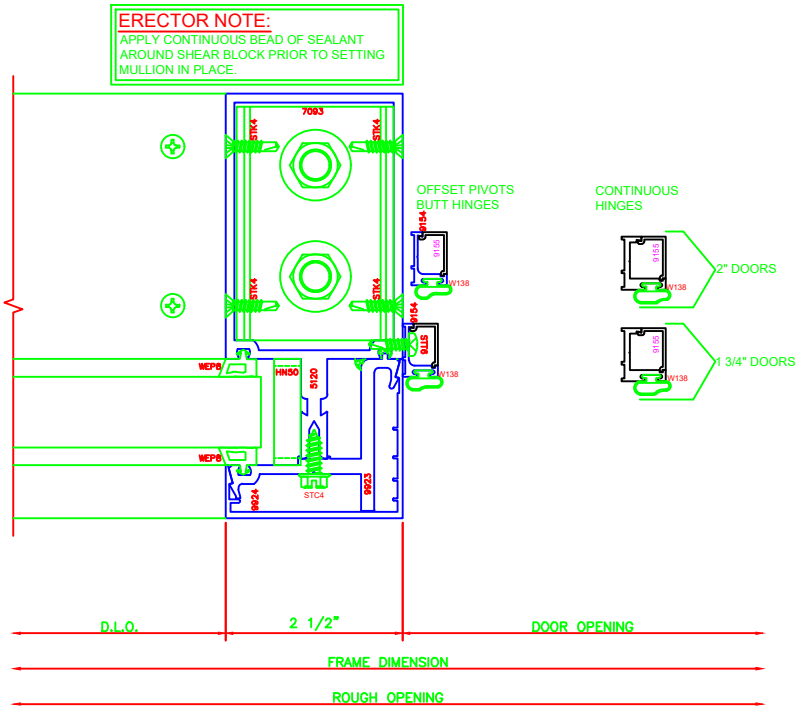
822 O.G. JAMB 5600 6"
